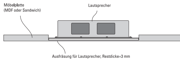
Schnitt DE Plan inside mit Ausfräsung
